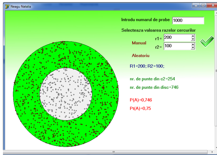
Fig. 3. Realizarea unui experiment din 1000 probe
