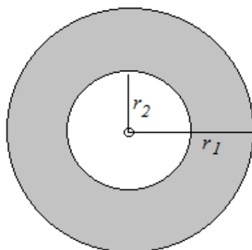
Fig. 1. Discul format de cercurile C_1 și C_2 .
