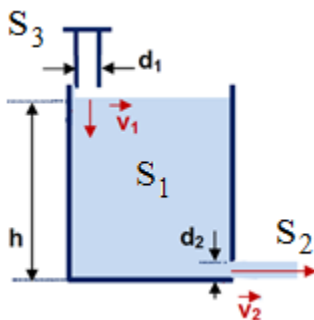
Figura 1. Conductă prin care curge apa într-un rezervor cu orificiu
